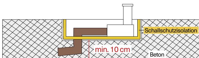
Ablaufanschluss senkrecht
