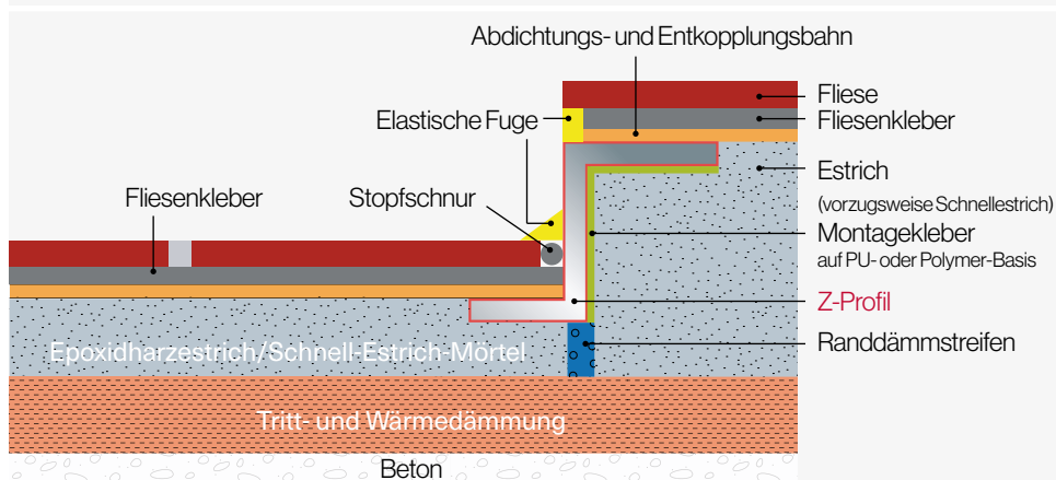
Z-Profil Typ ZR, ZL, ZRX u. ZLX
