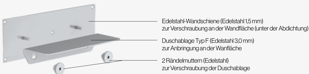
Einbauprinzip Duschablage Typ F (Flächenlösung)
