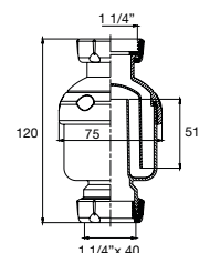
Siphon S-426, 1 1/4", 40 mm
