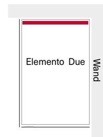
Ablaufkörper mit herausnehmbarem Siphon Sperrwasserstand 50 mm
