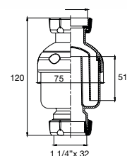
Siphon S-426, 1 1/4", 32 mm
