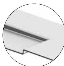
Z-Profil Typ ZRX und ZLX mit zusätzlich integriertem Schwallschutz
