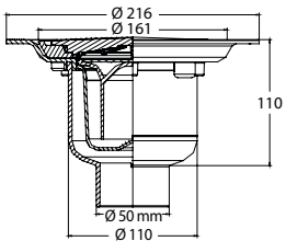
senkrecht
