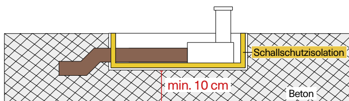
Ablaufanschluss waagrecht
