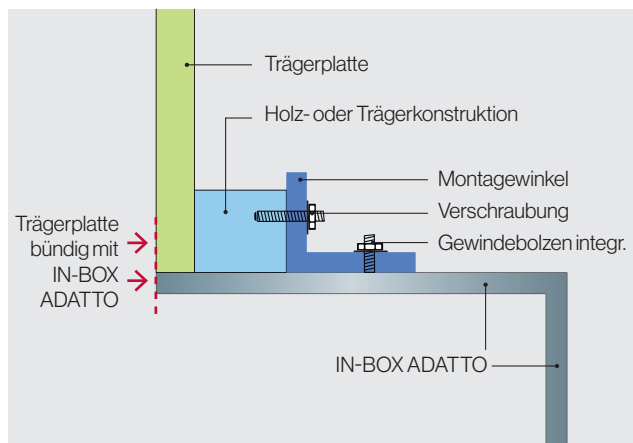
Prinzip Verschaubung mit Montagewinkel
