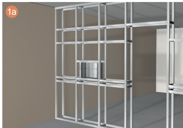
Die IN-BOX ADATTO in eine Holz- oder Trägerkonstruktion einpassen.
